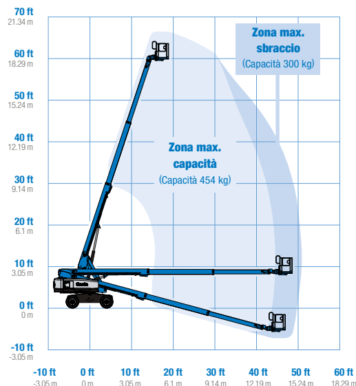
Diagramma di carico S-65 XC
