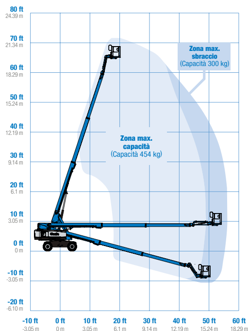
Diagramma di carico S-65 XC
